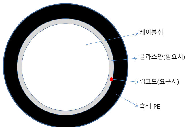
부도 3 세경 단일외장 광케이블의 외피구조
