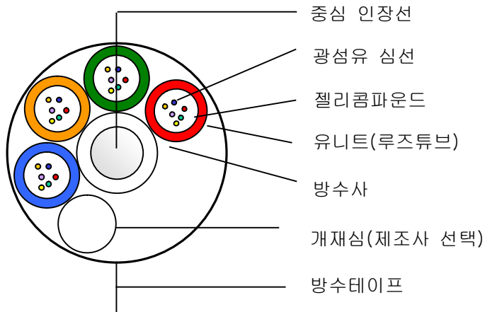
부도 3 세경 단일외장 광케이블의 외피구조
